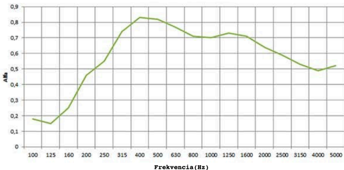
Graf činiteľa pohltivosti
