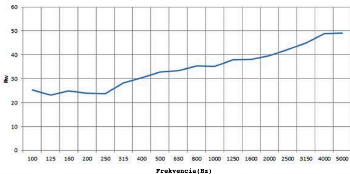
Graf laboratórnej vzduchovej nepriezvučnosti R_w : 35,3 dB
