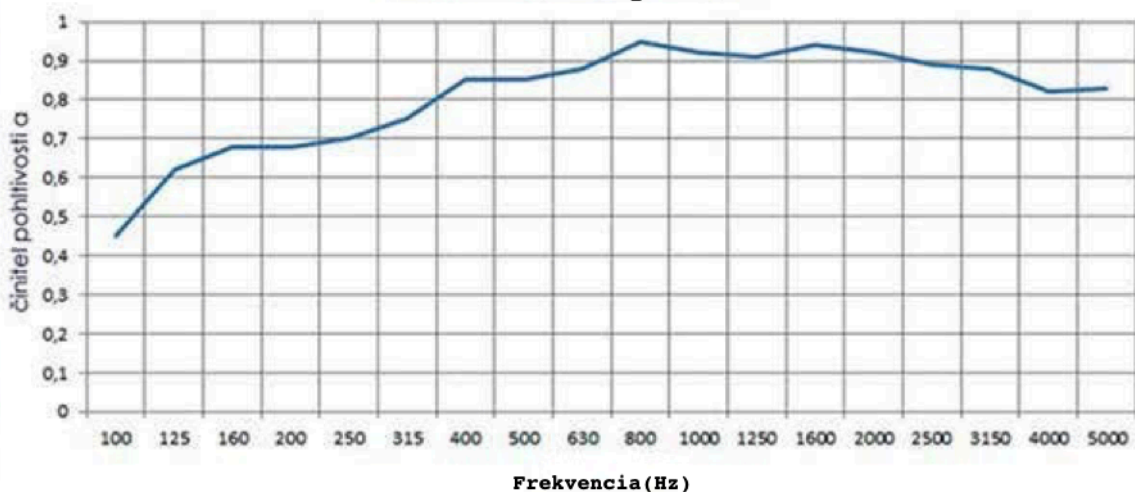
Graf činiteľa pohltivosti
