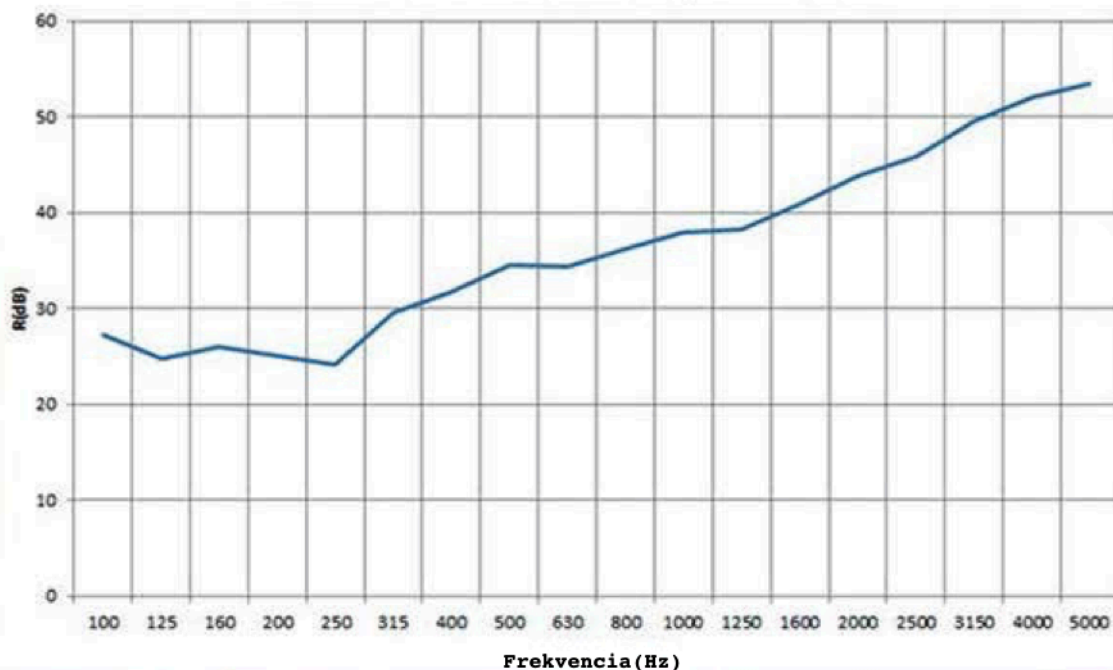
Graf laboratórnej vzduchovej nepriezvučnosti Rw: 37,0 dB
